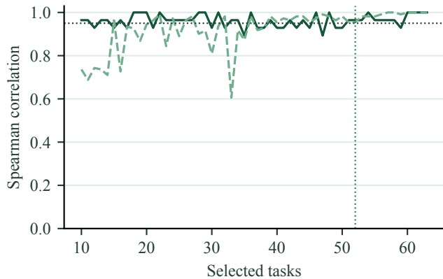
(d) OSWorld2 ranking
